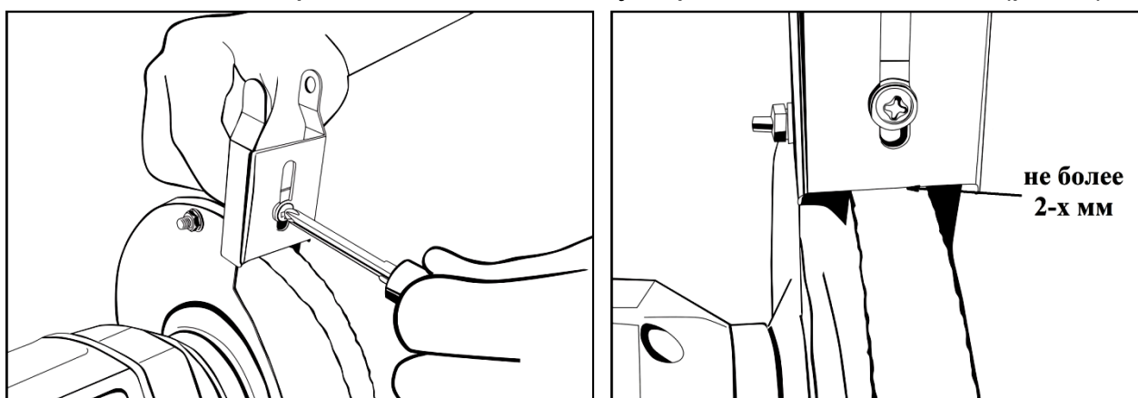
Рис. 2 «Установка искрогасителя» Рис. 3 «Регулировка искрогасителя»
